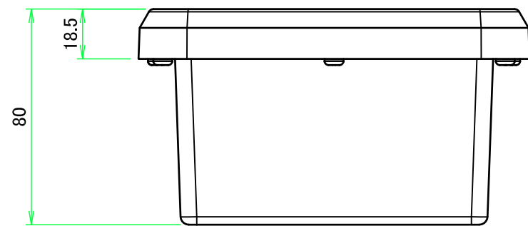
B-B ( 1 : 2 )
