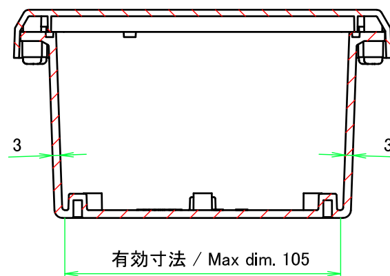
B-B ( 1 : 2 )
